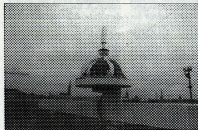
Šie ir vecais un jaunais mērinstruments, ar kuru mēra saules spīdēšanas ilgumu
