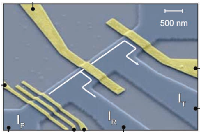
Gallija arsenīda nanostruktūra, kurā realizēts eksperiments. Baltās bultiņas izemē iespējamus elektronu ceļus.
